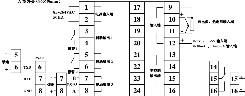
A 型外壳 (96×96mm)
